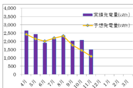
初号機～バンバン市民発電所～
