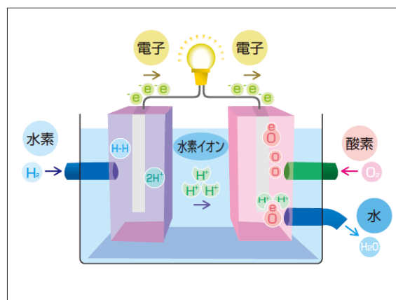
燃料電池の仕組み
