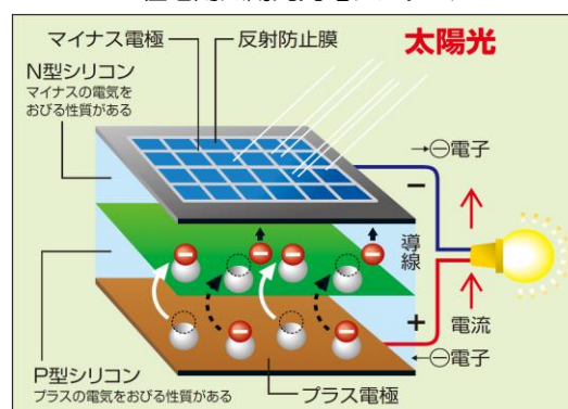
太陽光発電の仕組み
