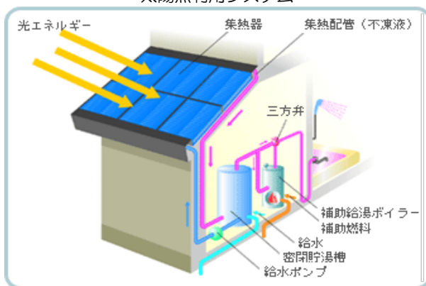
太陽熱利用の仕組み
