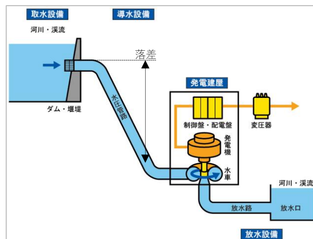
水力発電の仕組み
