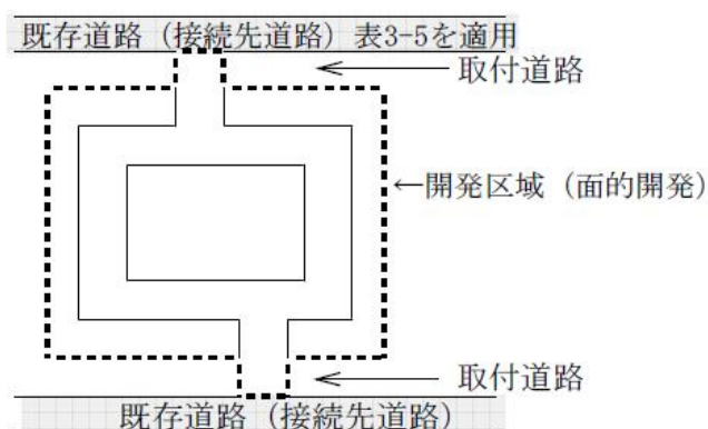
図3-5 接続道路
