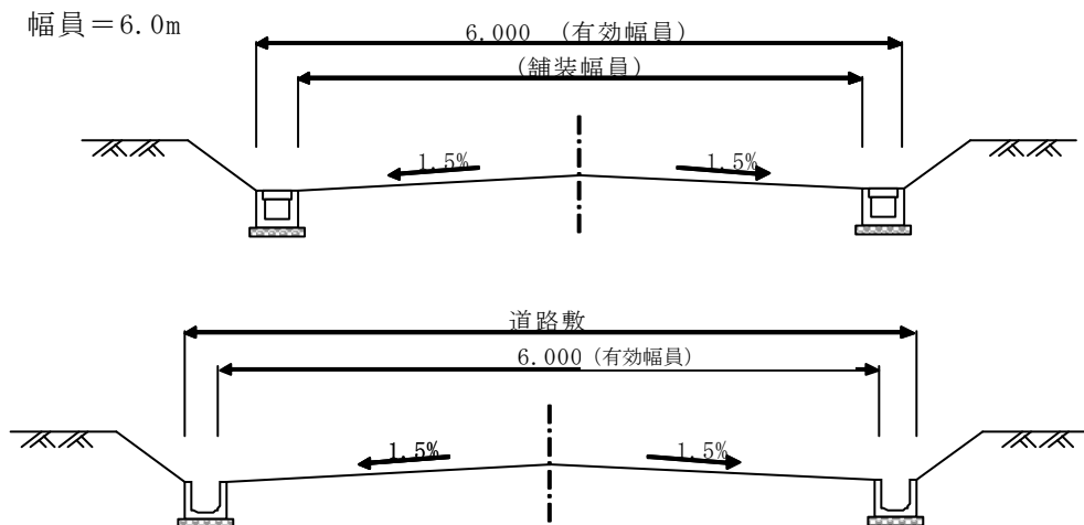
図 3-2 有効幅員のとらえ方
