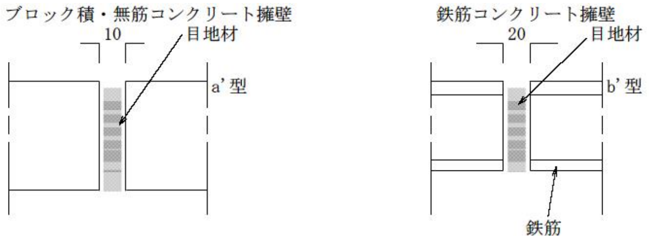
図 11-26 伸縮目地
