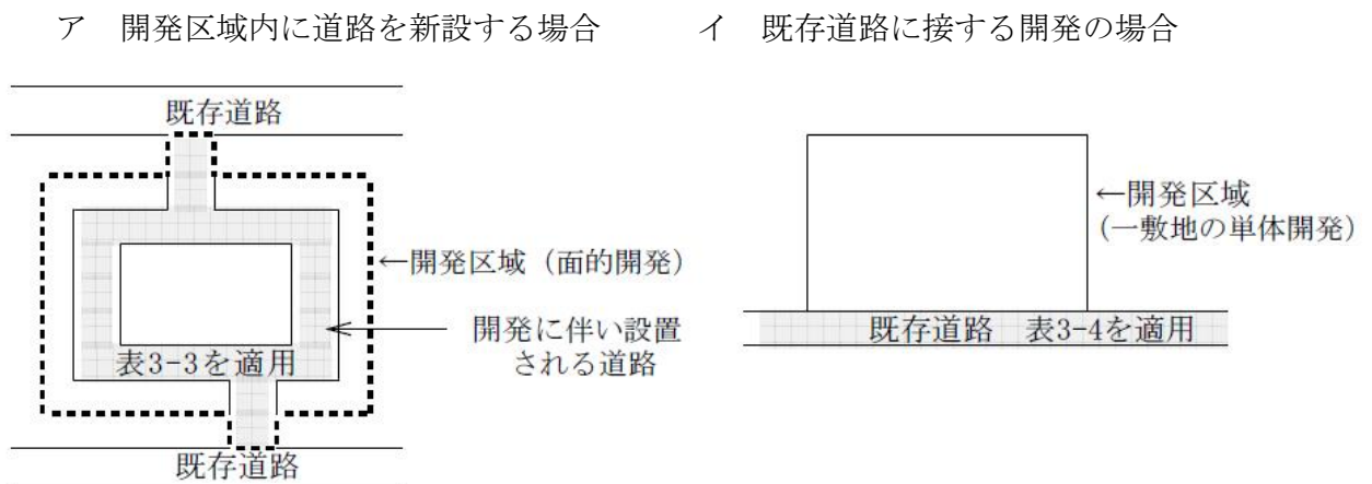
図 3-4 道路の幅員
