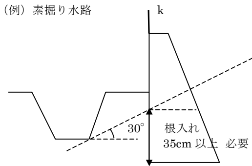
図 11-24 水路等に係る擁壁の根入れ
