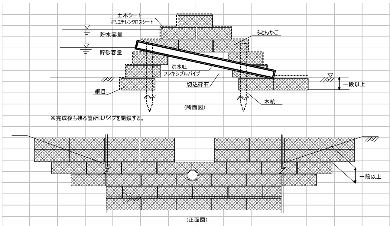
図 12—1 小規模な仮の防災調整池の例
