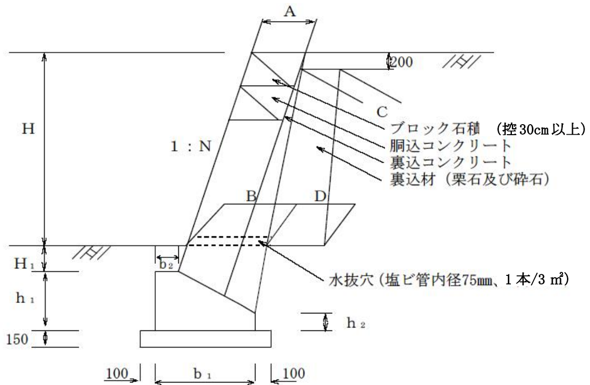
図 11-16 練積み造擁壁の構造
