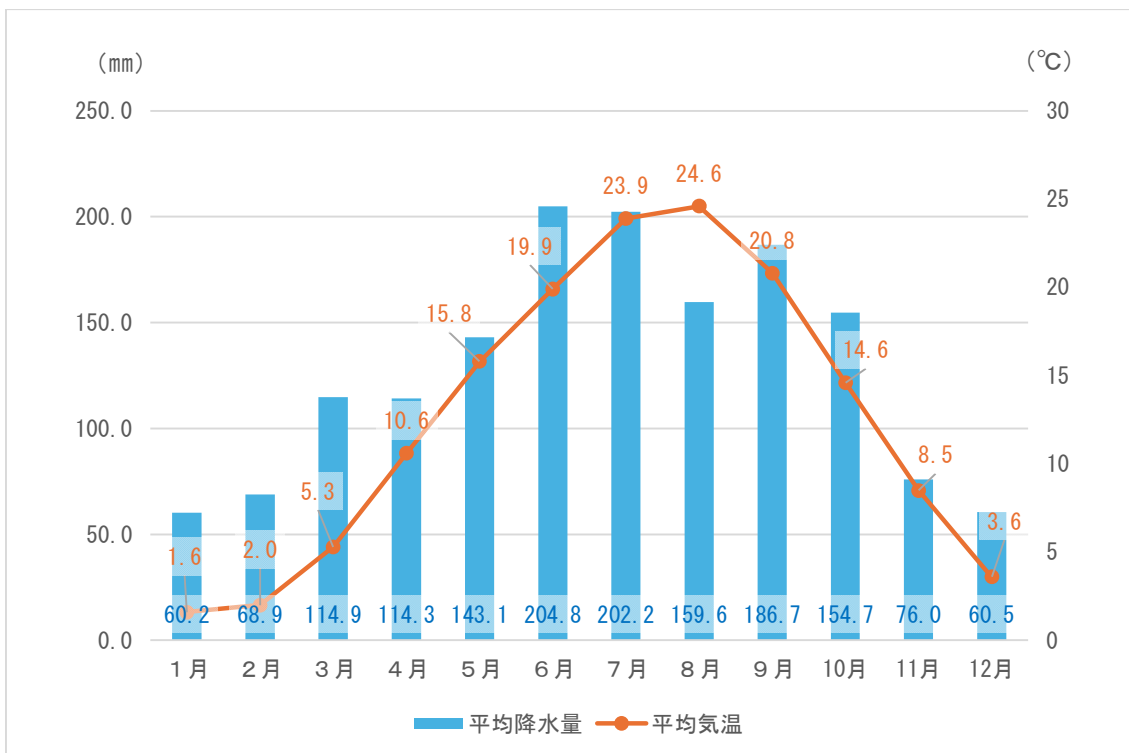
21 図7 本市の年間平均降水量と年間平均気温
