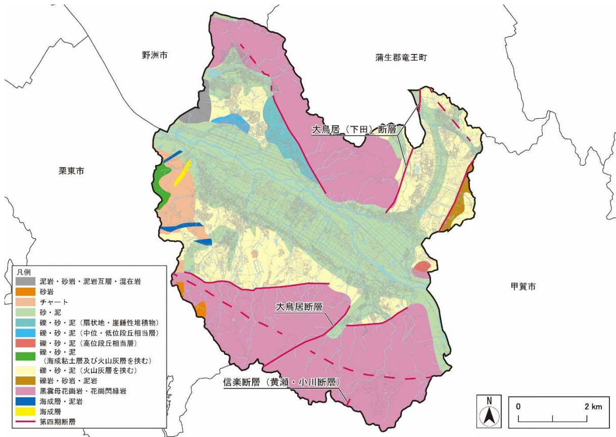
29 図 6 本市の地質図
