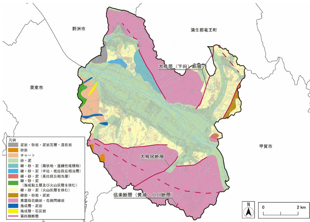
図6 本市の地質図
