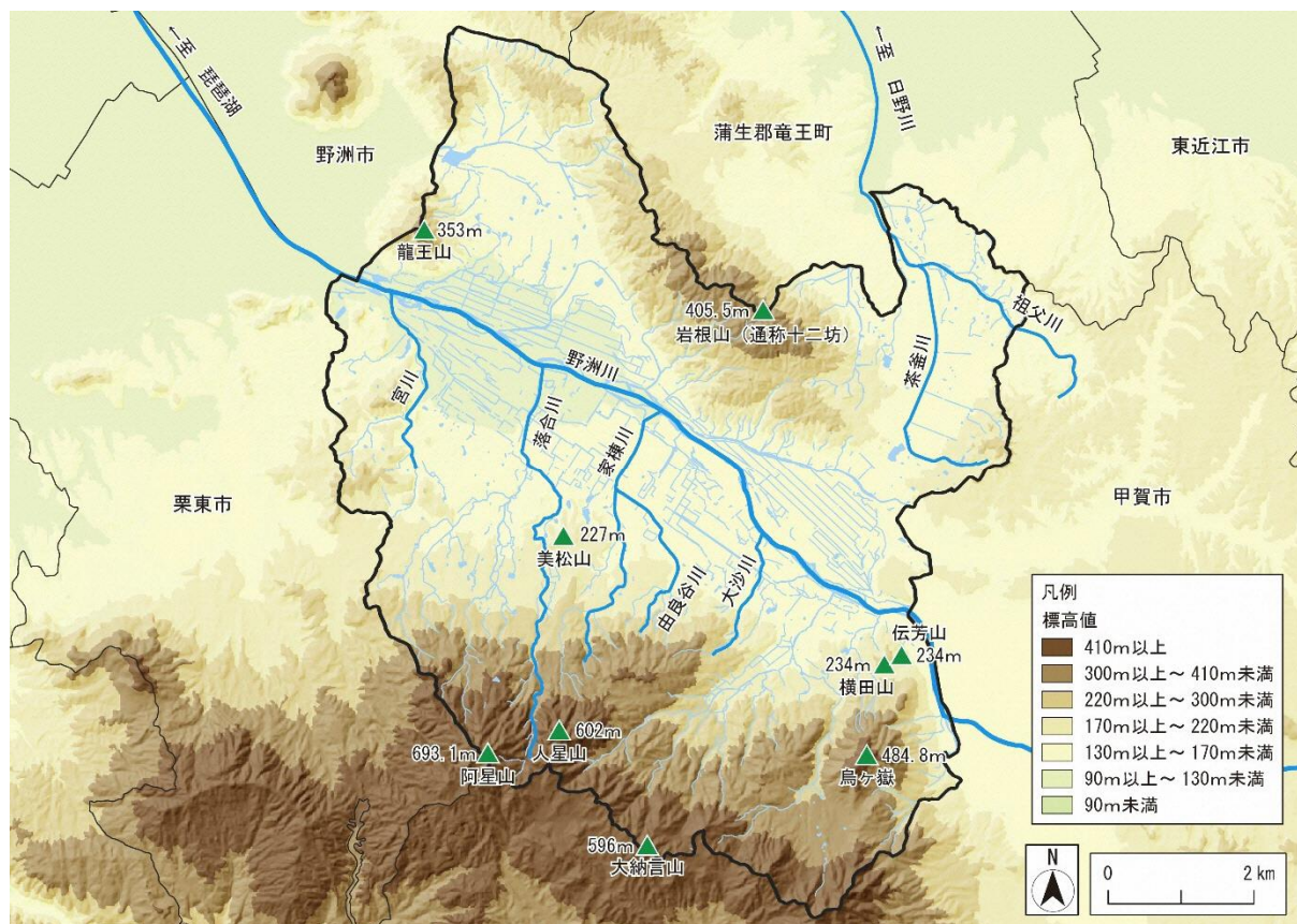
図5 本市の地形図
