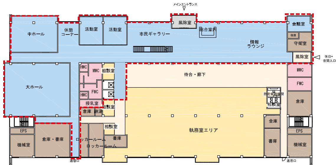
1階平面図
