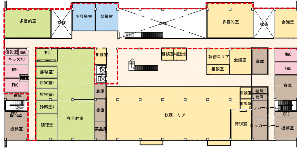
2階平面図
