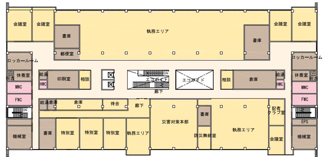
3階平面図
