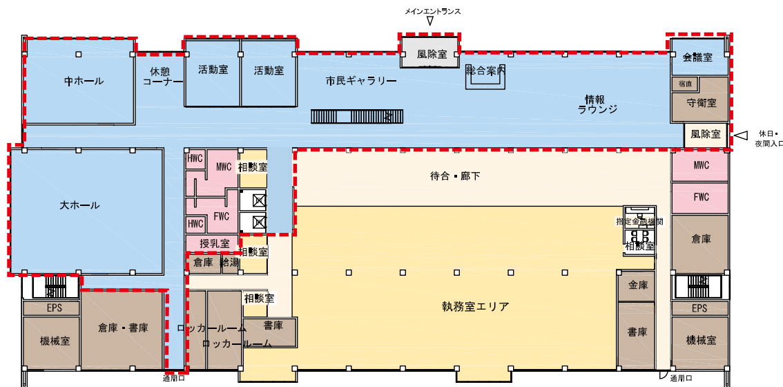
1階平面図
