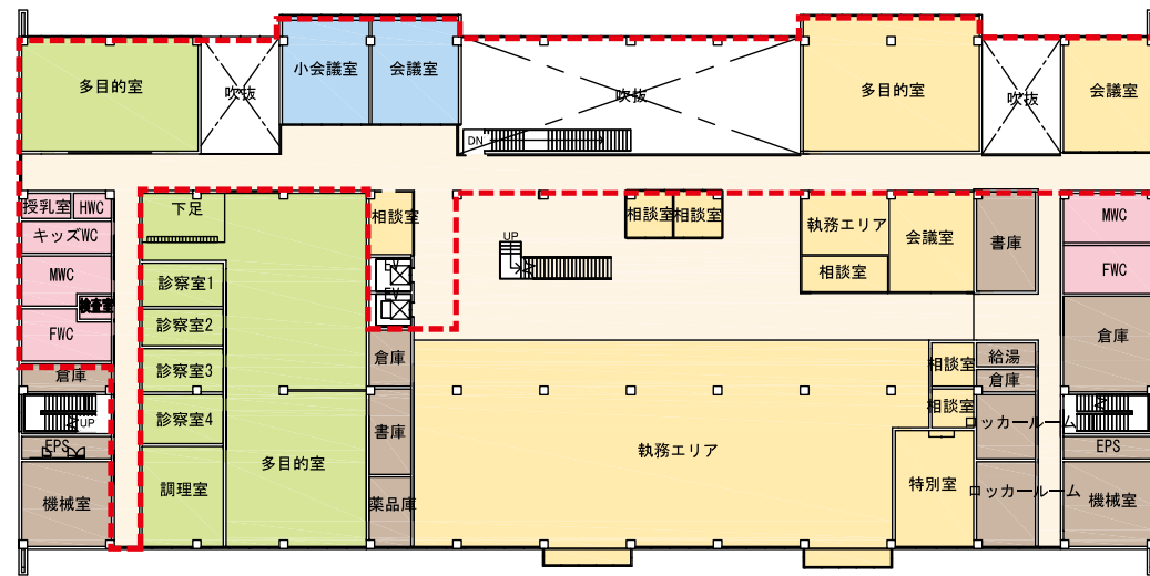
2階平面図
